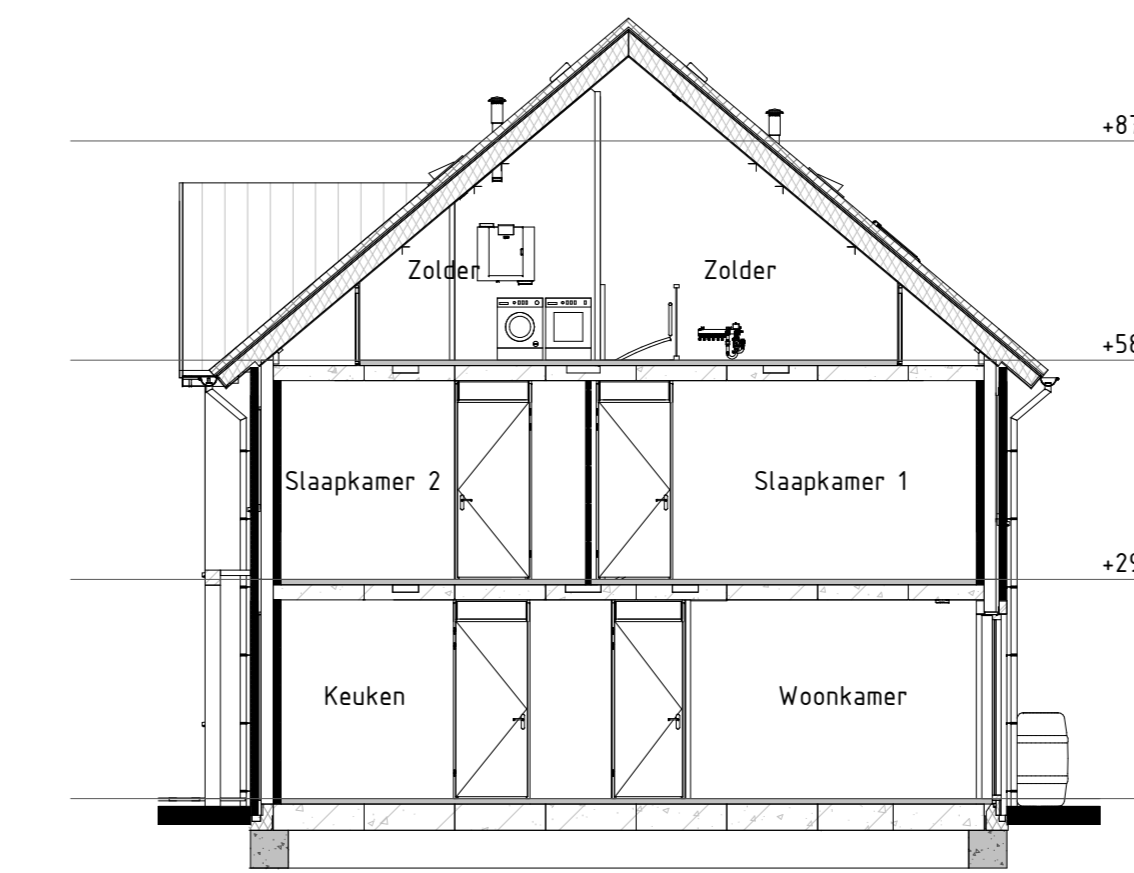
Dwarsdoorsnede
