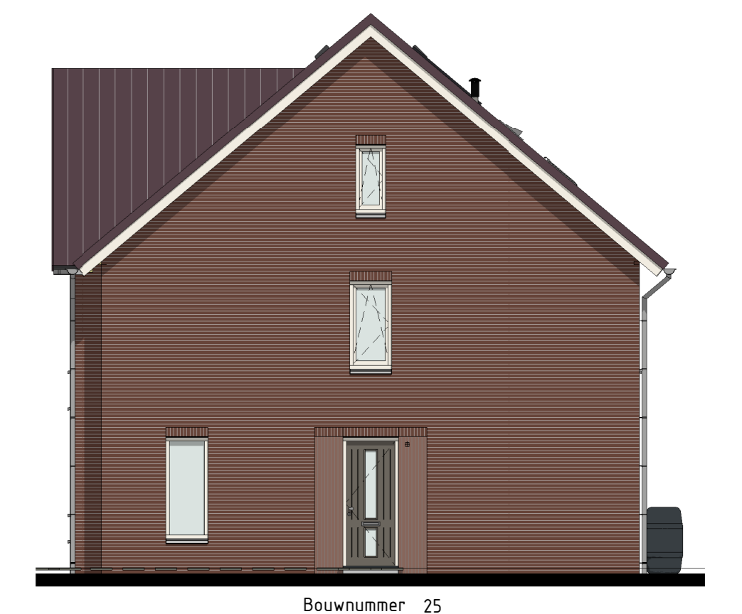
Rechtergevel
