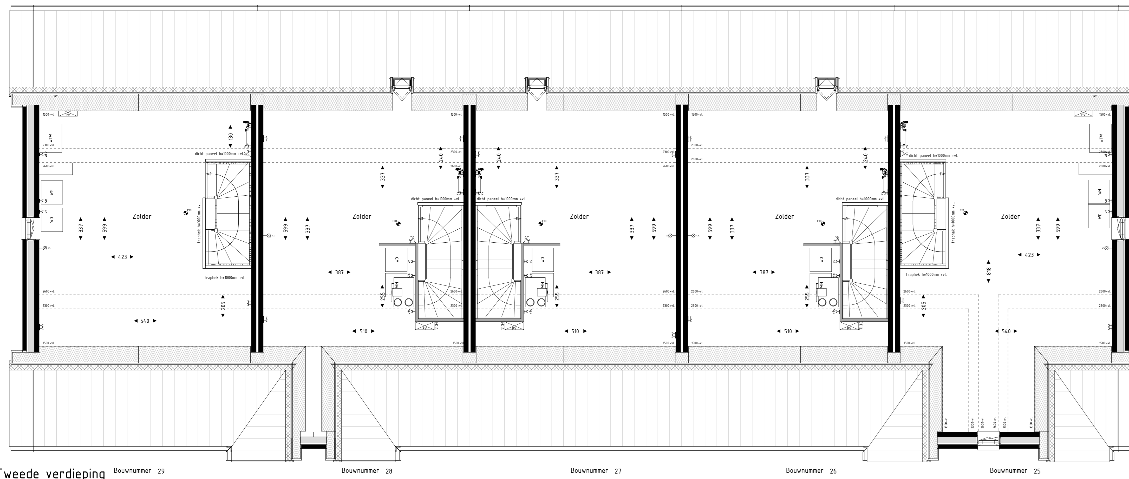
Tweede verdieping
