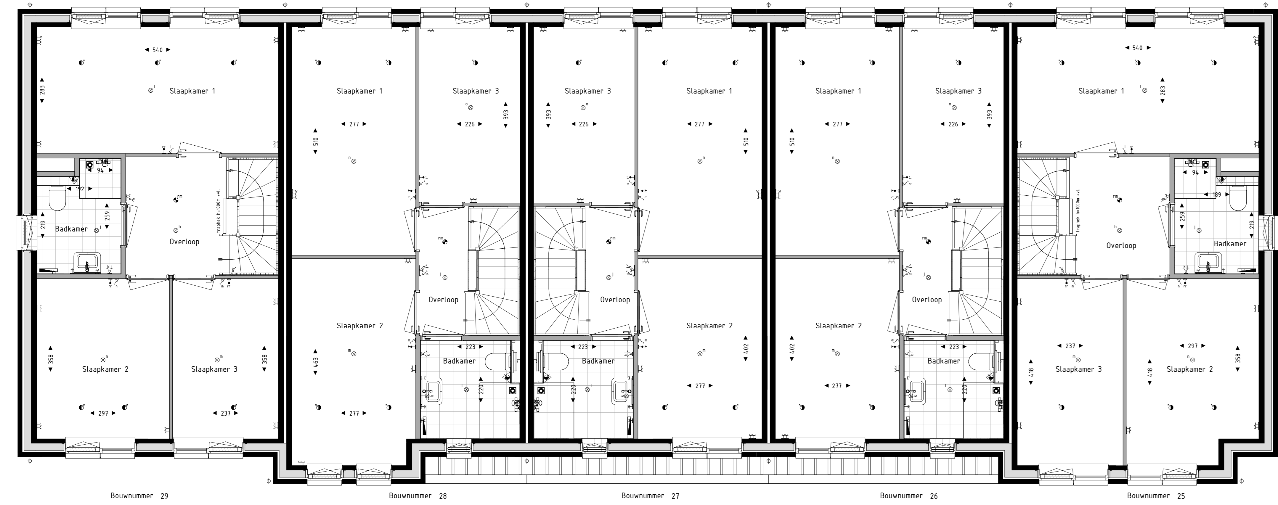
Eerste verdieping
