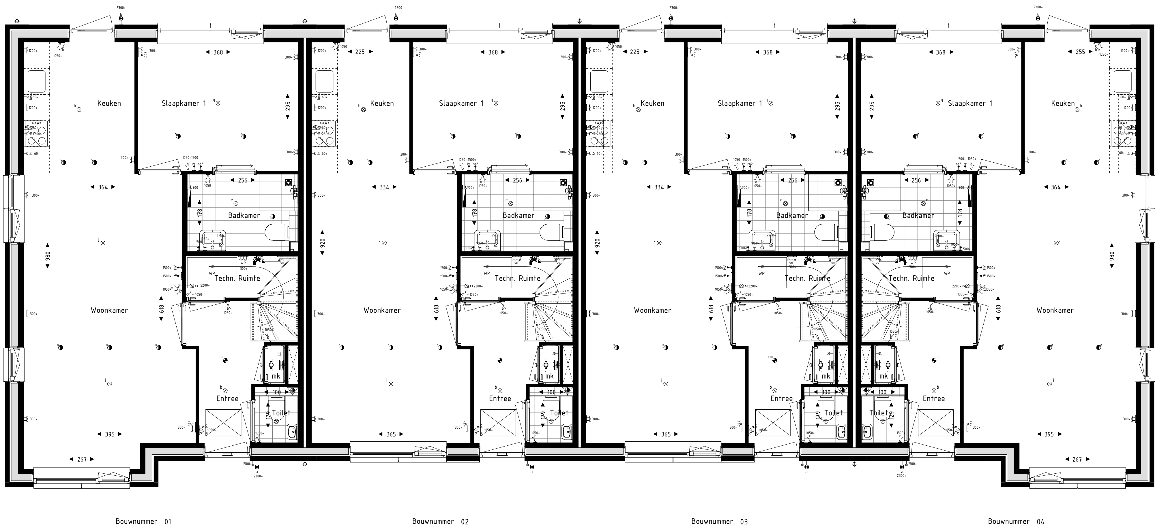
Begane grond
