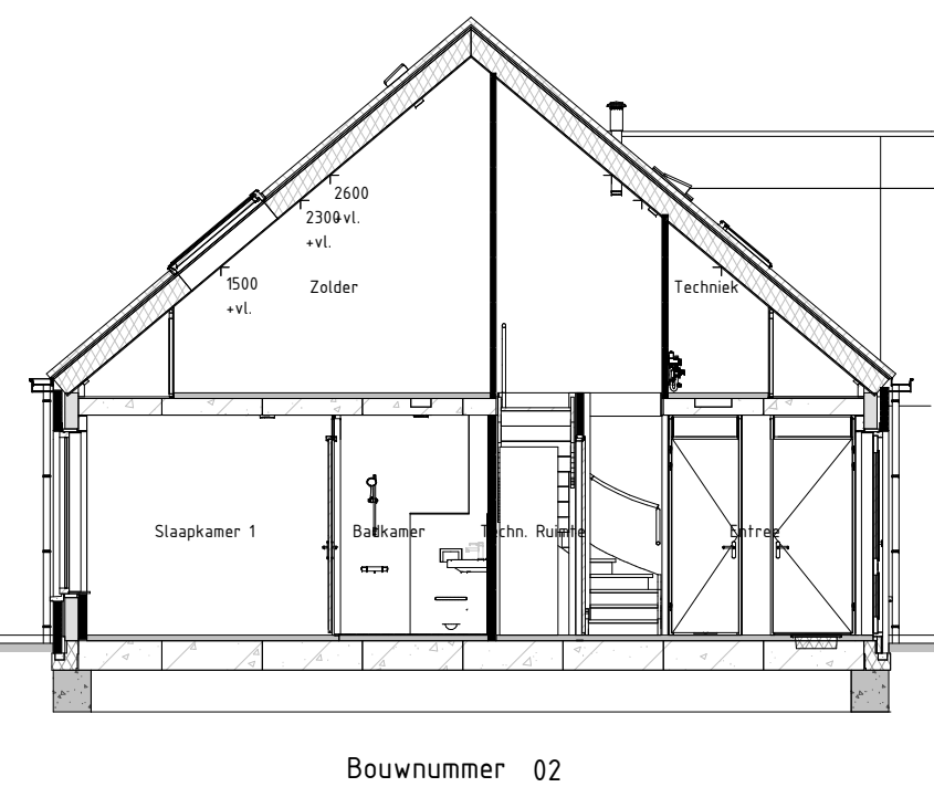
Doorsnede AA
