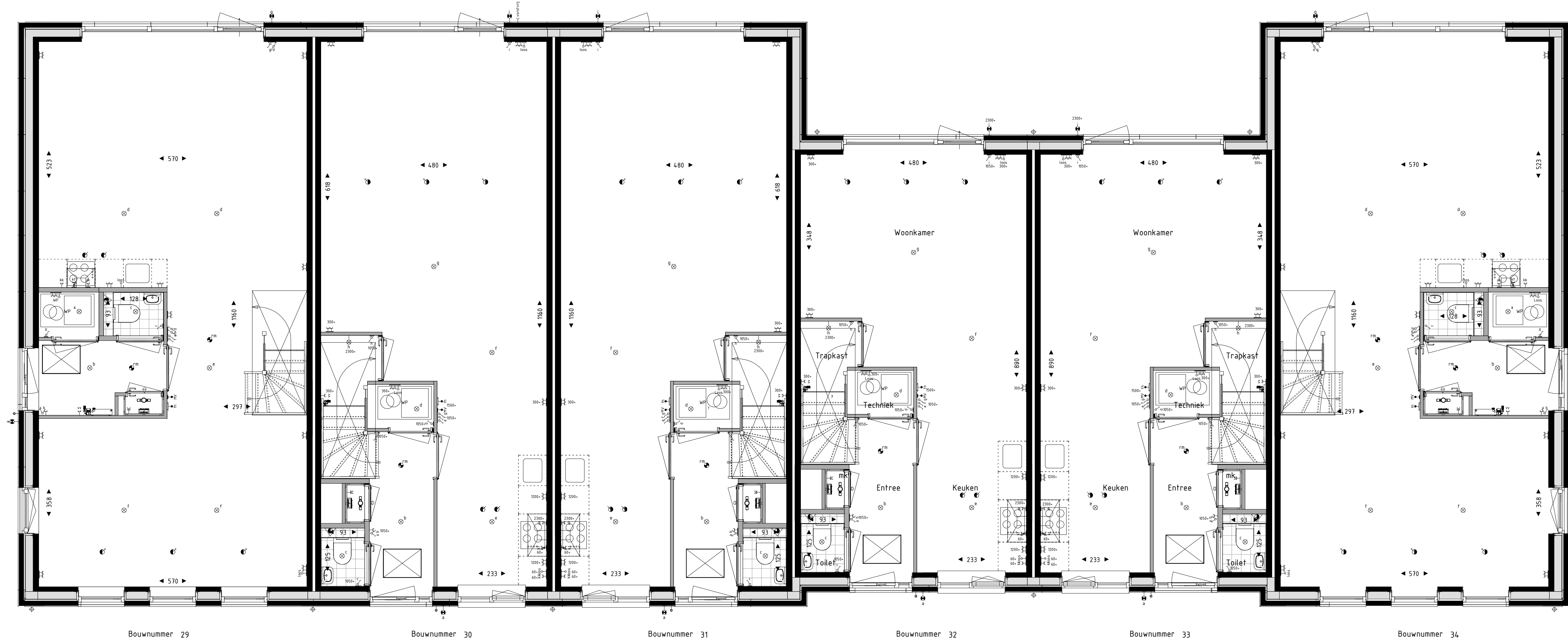
Begane grond
