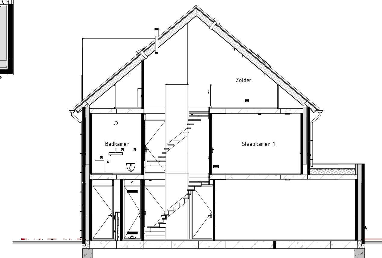
Dwarsdoorsnede
